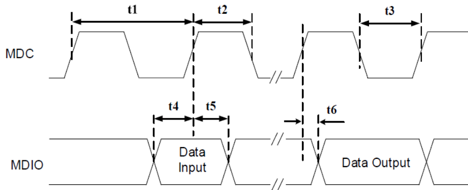
Figure 14. SMI (MDC/MDIO) Timing
